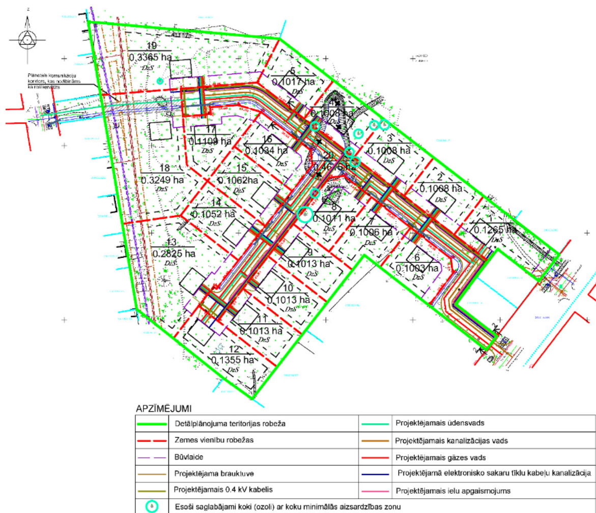
Attēls Nr. 8. Inženierkomunikāciju shēma.
