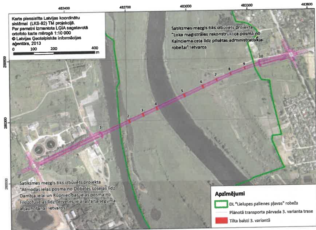
3. attēls. 3. alternatīvas tilta balstu vietas
